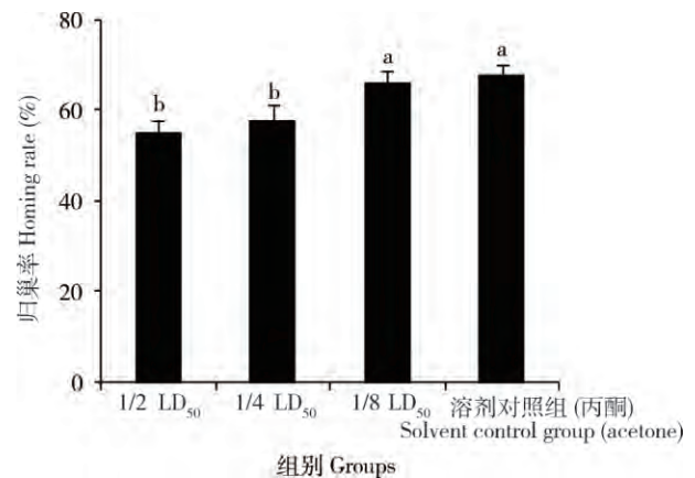
图3 不同浓度高效氯氟氰菊酯对西方蜜蜂工蜂归巢能力的影响
