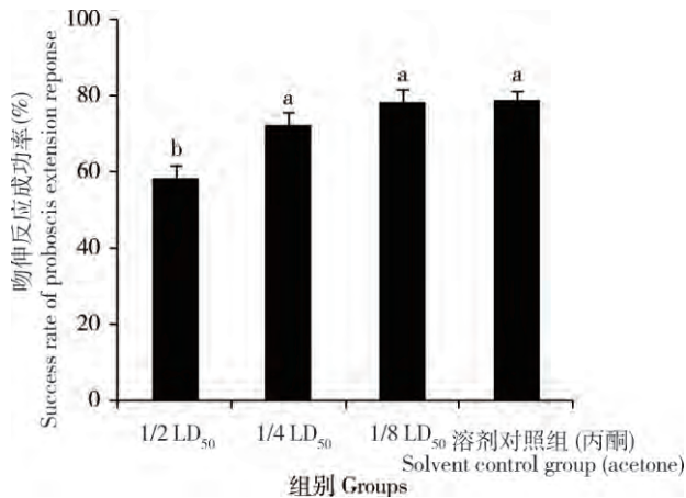
图2 不同浓度高效氯氟氰菊酯对西方蜜蜂工蜂学习记忆能力的影响
